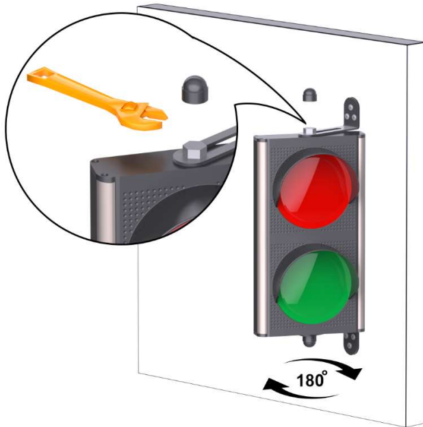
Şekil 4.3 – TRFL sabitleme ve somunların kapanması.
