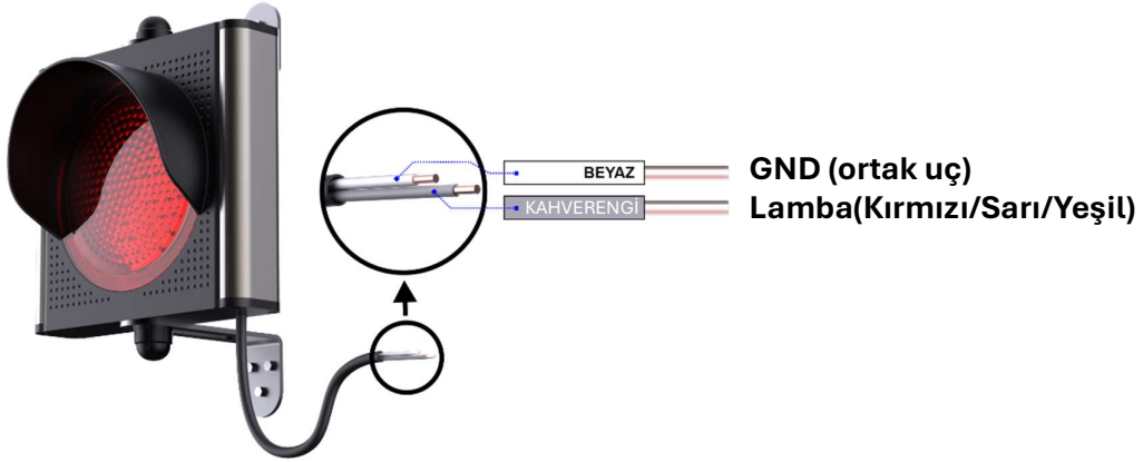
Şekil 3.1 - TRFL1 Bağlantı Şeması
