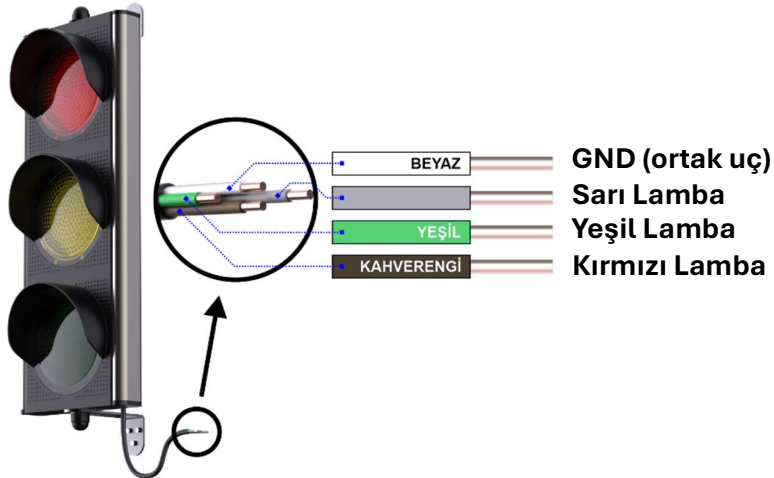
Şekil 3.3 – TRFL3 Bağlantı Şeması
