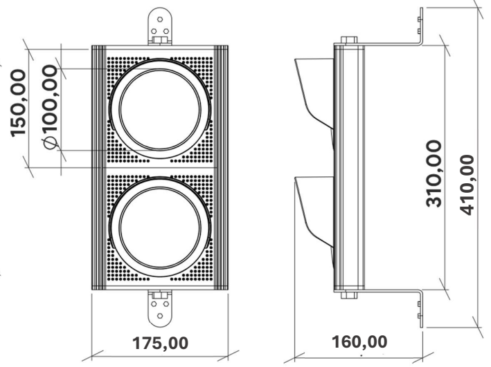
Ölçü Birimi: mm Şekil 4.5 – TRFL2 ölçüleri.
