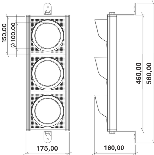
Ölçü Birimi: mm Şekil 4.6 – TRFL3 ölçüleri.
