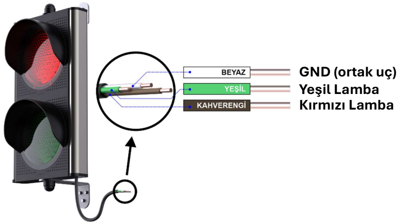
Şekil 3.2 – TRFL2 Bağlantı Şeması
