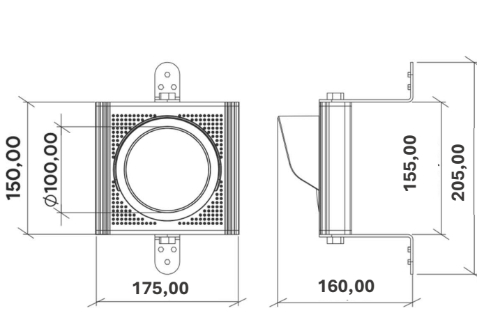
Ölçü Birimi: mm Şekil 4.4 – TRFL1 ölçüleri.
