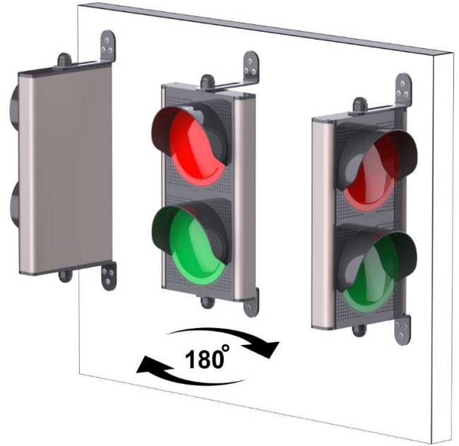
Şekil 4.2 – TRFL açı ayarı.
