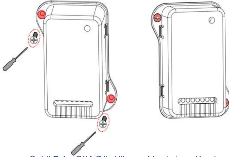
Şekil 7.1 – RKA Düz Yüzeye Montajının Yapılması
