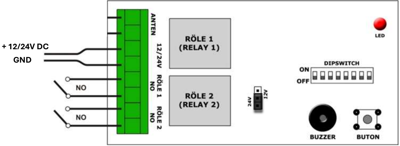
Şekil 8.1 RKA/RKA2 Bağlantı Şeması
