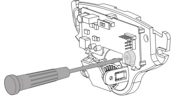
Şekil 6.4 RDR2 Çalışma ayarlarının yapılması.
