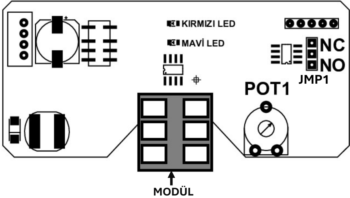
Şekil 4.1 RDR2 Kontrol Kartı
