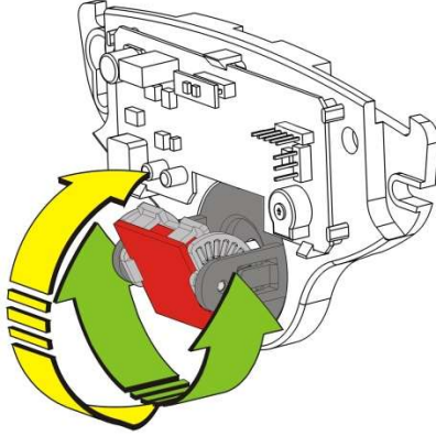
Şekil 6.3 RDR2 Algılama açısının ayarlanması.
