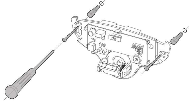
Şekil 6.2 RDR2 Duvar montajı yapılması.
