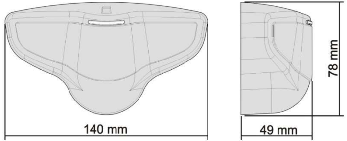
Şekil 6.6 RDR2 boyutlar birim mm.
