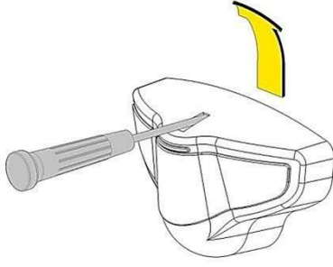
Şekil 6.1 RDR2 Üst kapağın sökülmesi.
