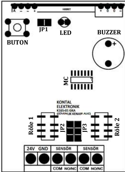
Şekil 2 - Güvenlik Kenarı Alıcısı (GKA)
