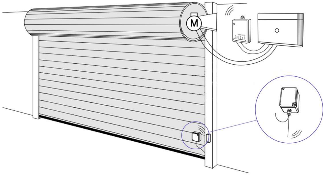
Şekil 7 - Kepenklerde Kullanım
