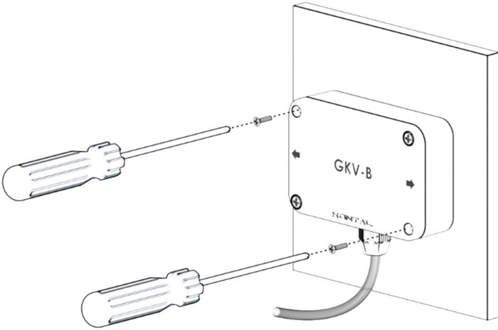
Şekil 15 – GKV-B Üst Kapak Montajı
