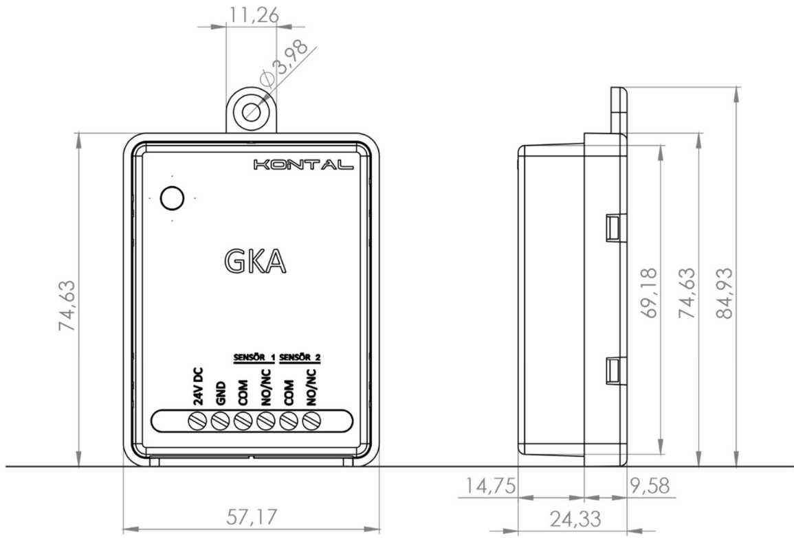
Şekil 16 - GKA Boyutlar
