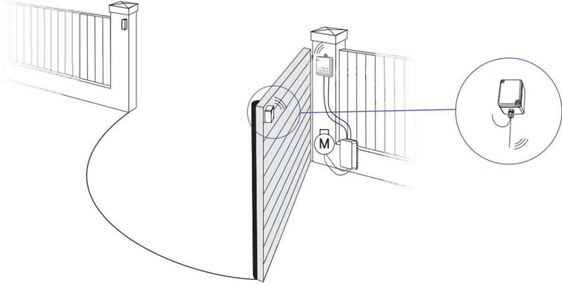
Şekil 8 - 90° Bahçe Kapılarında Kullanım
