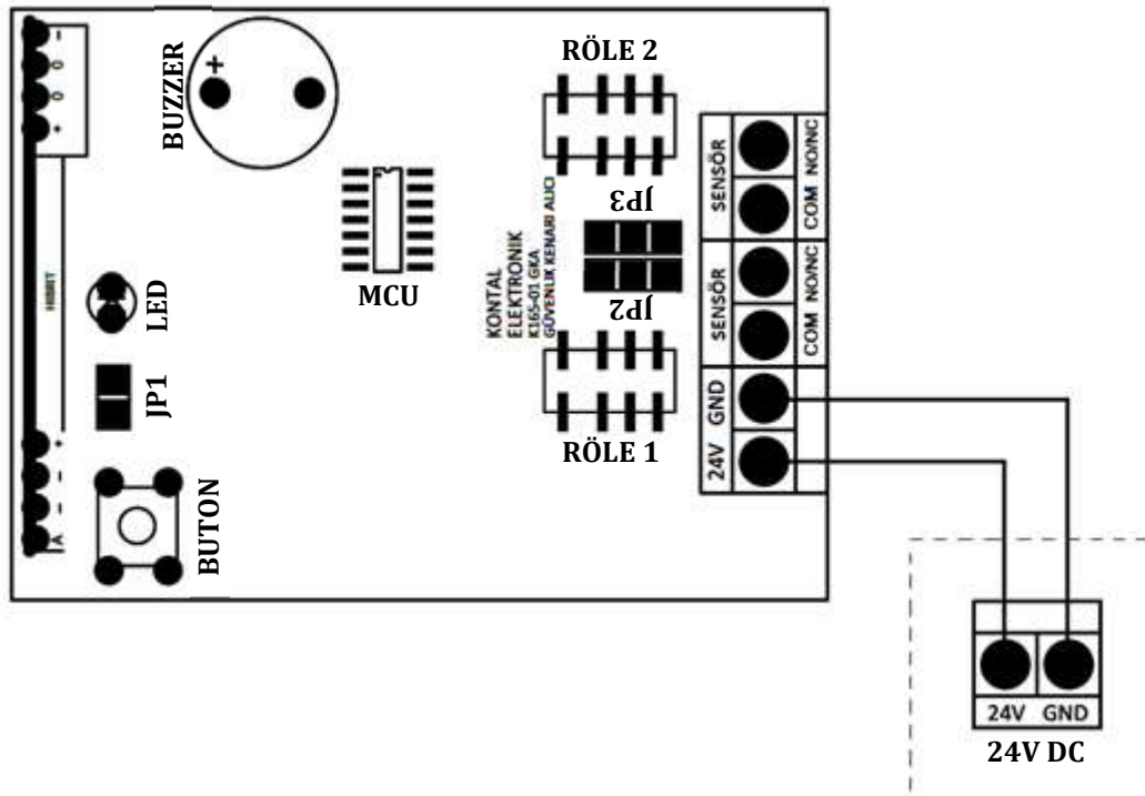
Şekil 12 - GKA Bağlantı Şeması
