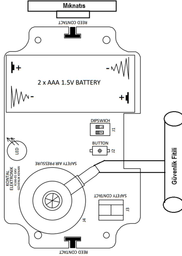
Şekil 11 – GKV-B Bağlantı Şeması
