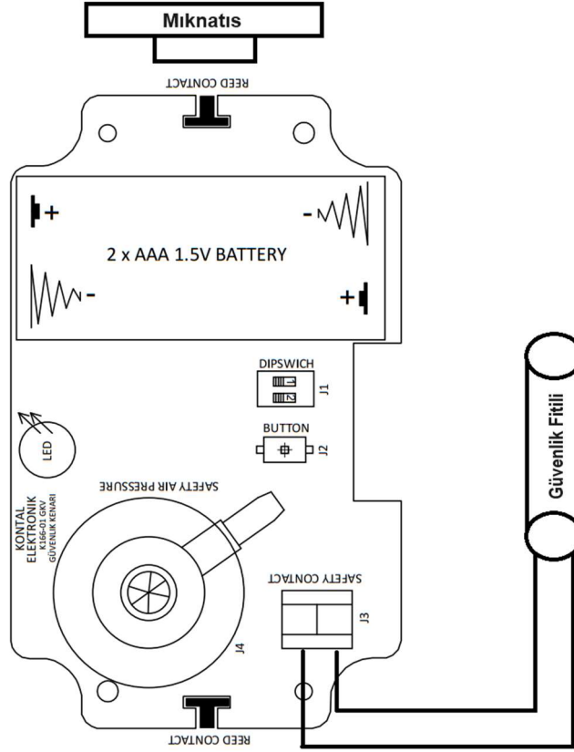
Şekil 11 – GKV Bağlantı Şeması
