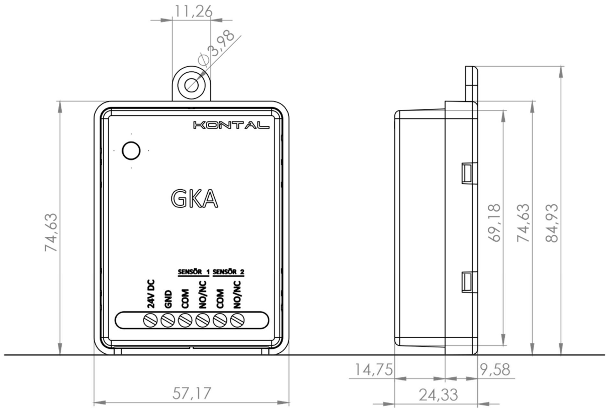
Şekil 16 - GKA Boyutlar
